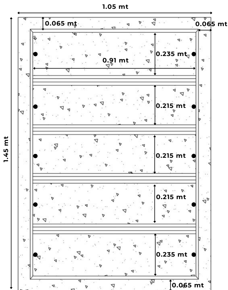
Vista frontal Escala gráfica
