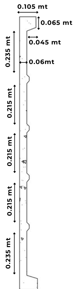
Corte placa Escala gráfica
