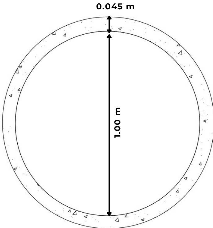
VISTA SUPERIOR - ARO PARA POZO Escala gráfica
